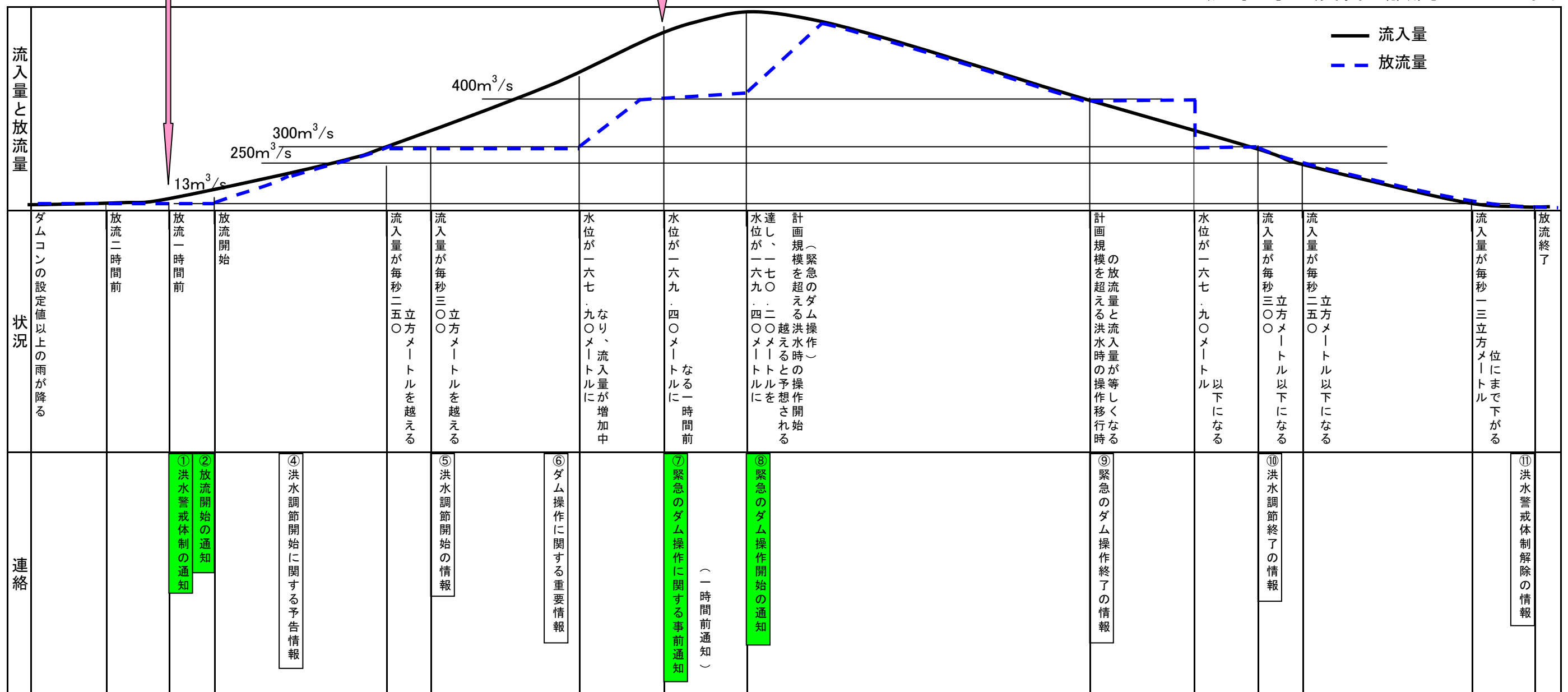
洪水対応演習 放流イメージ図
