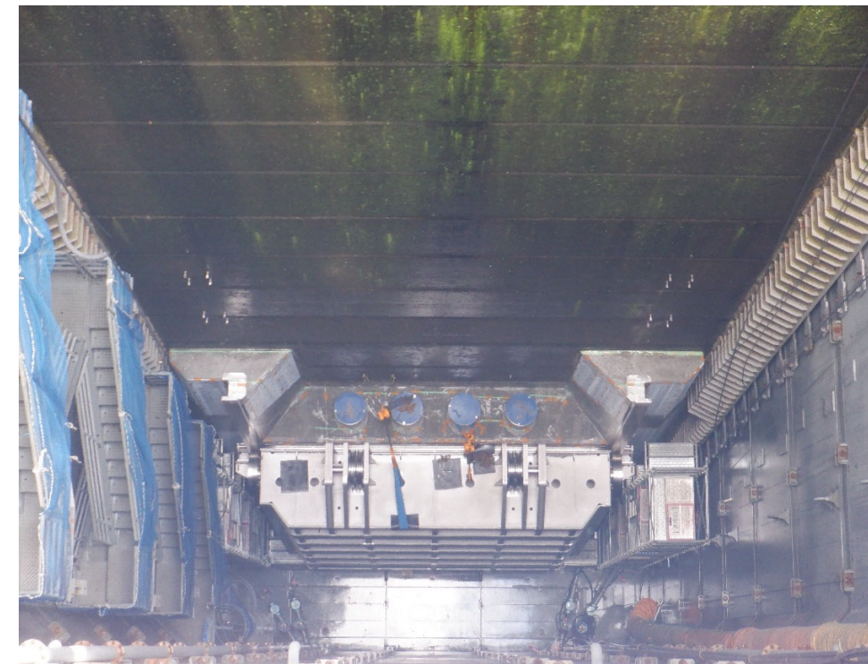
堤体上流面 予備ゲート設置状況
