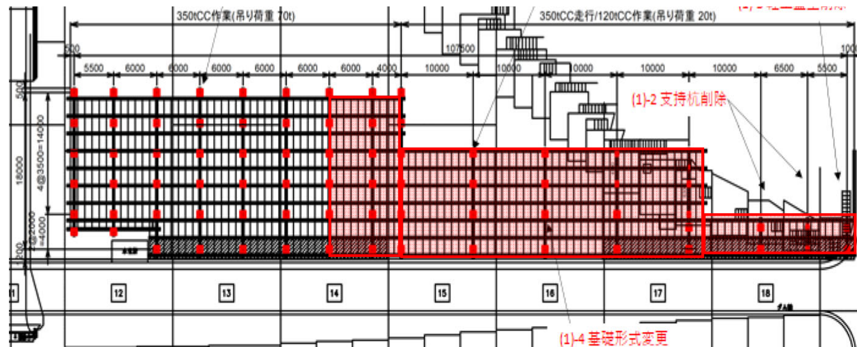
天端仮設構台 (地組・設置)
