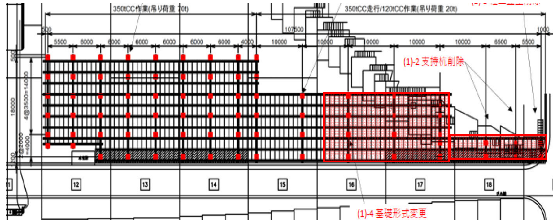
天端仮設構台 (地組・設置)
