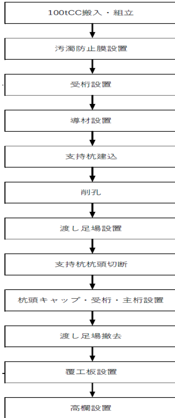
施工フロー図
