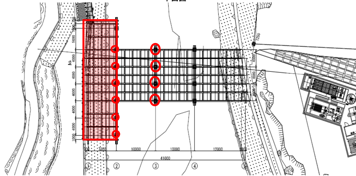
渡河橋一般図 平面図
