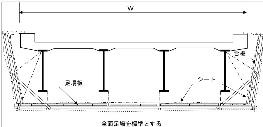
パイプ吊足場参考図
