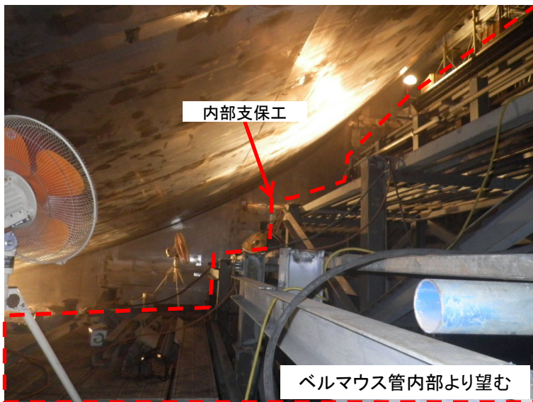
7月3日 ベルマウス管内部支保工(上流部)撤去
