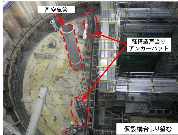
7月24日 副空気管・戸当り設置
