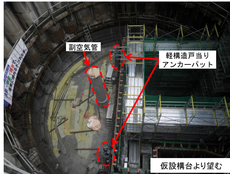
7月10日 副空気管・戸当り設置
