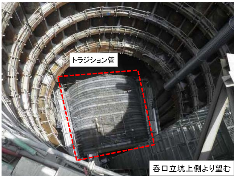
5月23日 トランジション管溶接完了
