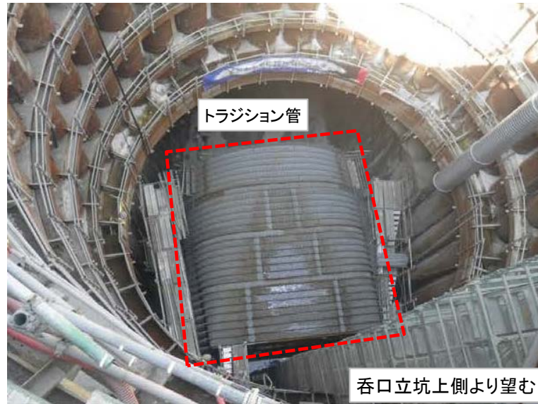
5月16日 トランジション管溶接
