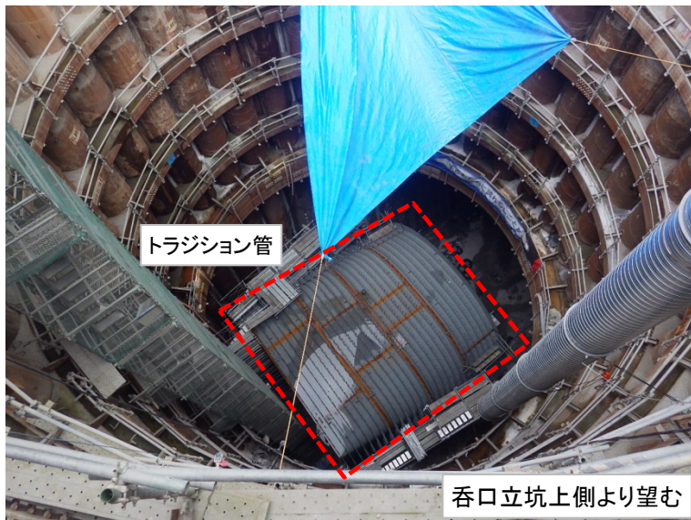
5月9日 トランジション管溶接
