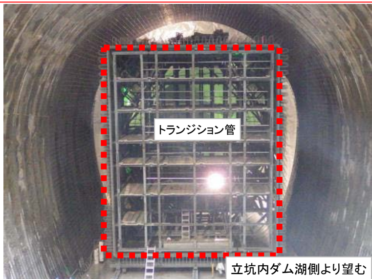
6月6日 トランジション管据付固定
