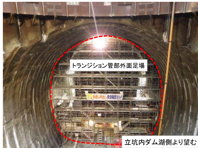
6月27日 鋼製埋設型枠設置(3リフト目)
