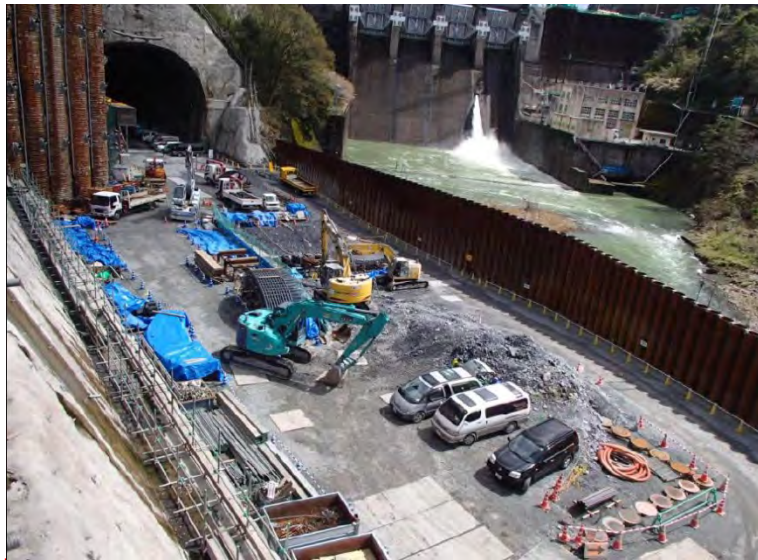
4月7日 トンネル工準備作業
