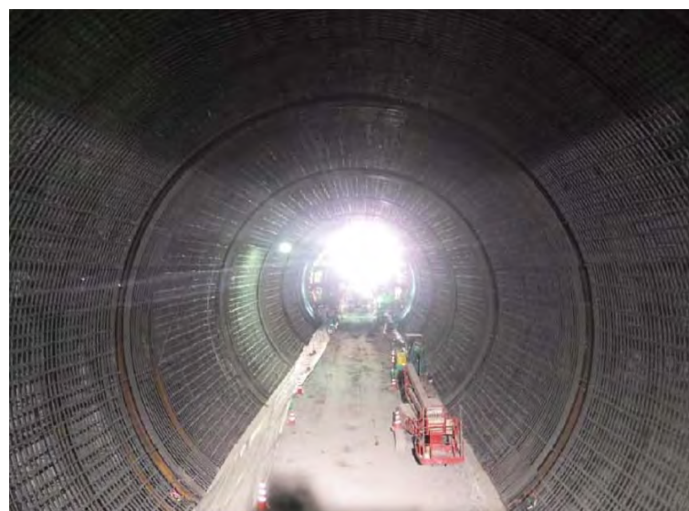
4月14日 インバート工、覆工
