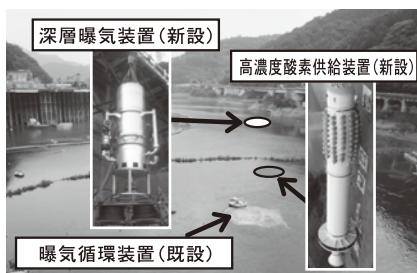
【ダム堰堤から見た各施設の位置】
