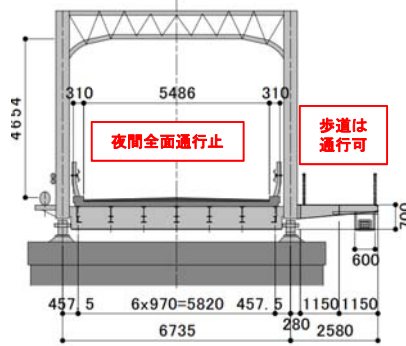
橋梁諸元
