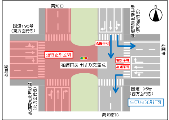
布師田あけぼの交差点通行止め詳細
