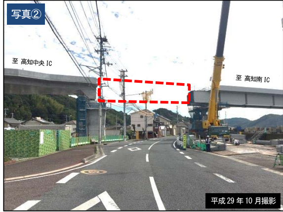
橋梁架設箇所
