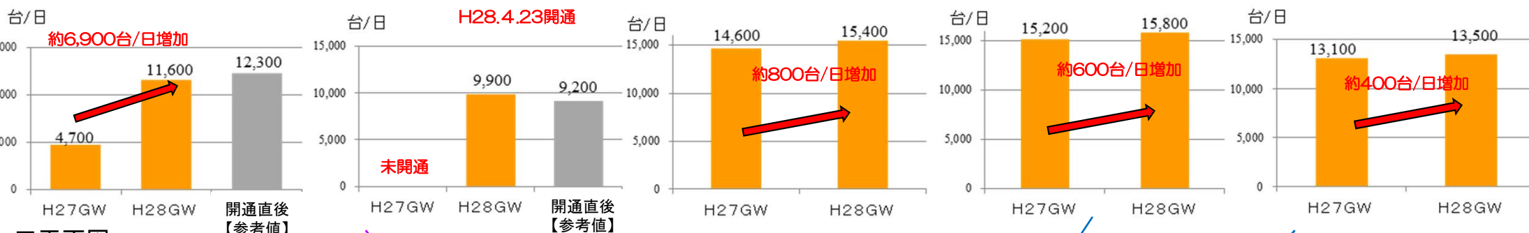
断面① 高知南国道路 (高知南IC～なんこく南IC)
