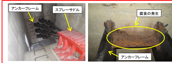
【アンカーレージ】 スプレー室内の雨水浸入による滞水及びアンカーフレーム等の腐食
