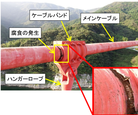
【メインケーブルカバーの腐食破断状況】
