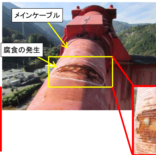
【メインケーブルカバーの腐食状況】
