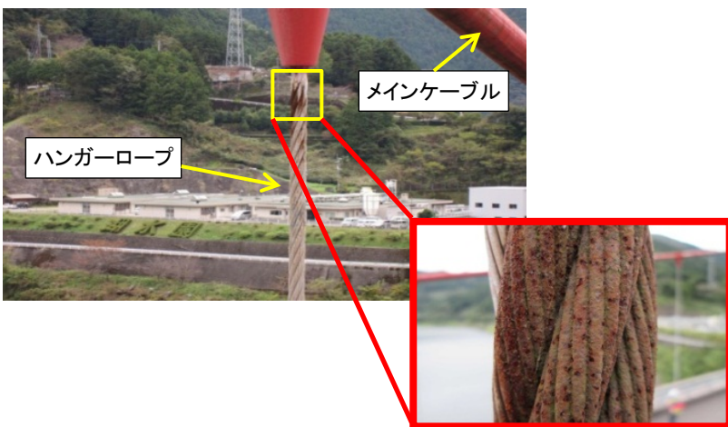
【ハンガーロープの腐食状況】
