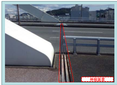
伸縮装置の損傷状況
