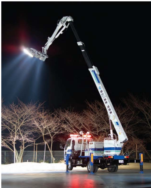
強力な照明装置を搭載している照明車
