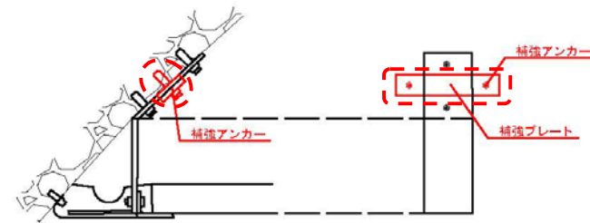
面端支持金具補強イメージ (A部)
