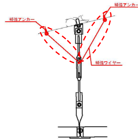
天井板吊金具補強イメージ (B部)
