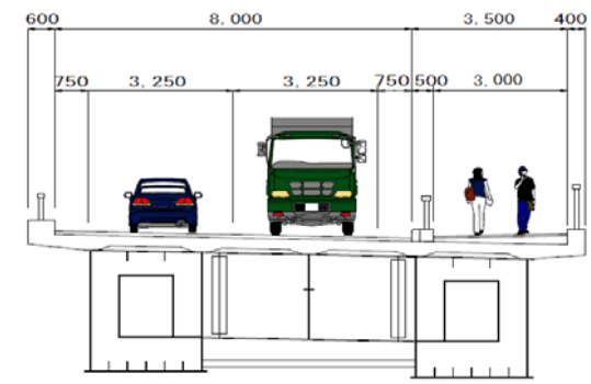
<暫定型(橋梁部)>
