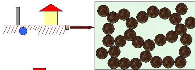
じばん 地盤 のなりたち
