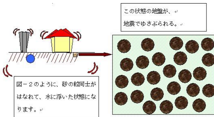
じばん 液状化した地盤
