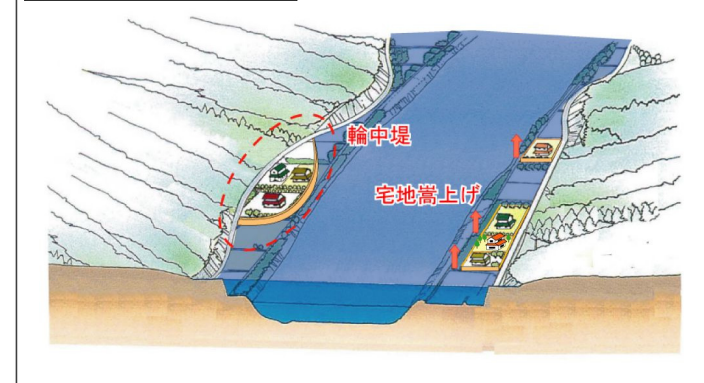
図－4.1.2 輪中堤・宅地嵩上げ等の整備イメージ
