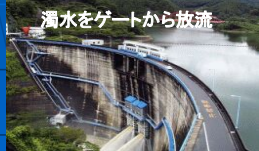
放流設備追加後: 濁度分を洪水中に放流
