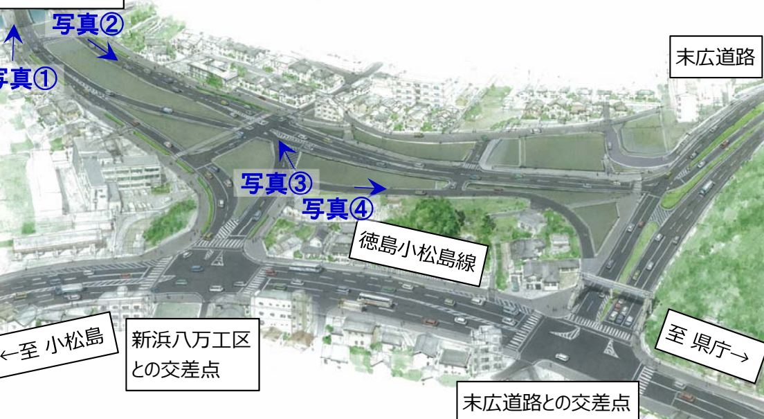
新浜八万工区 【②「末広道路」と「新浜八万工区」を直結する暫定的な道路整備】パース図
