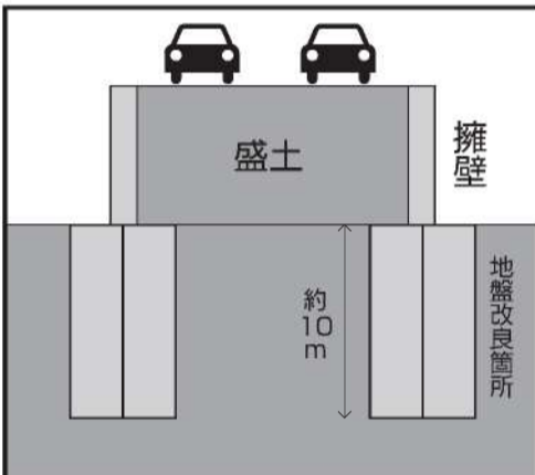
右の計画予定写真で紹介している道路の断面図。
