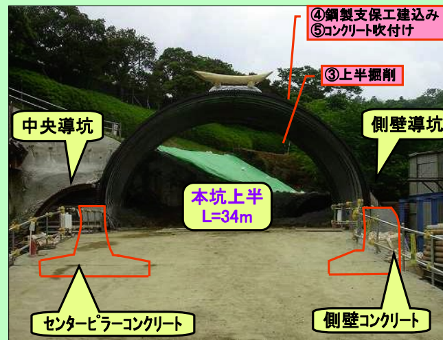
トンネル坑口(入り口)
