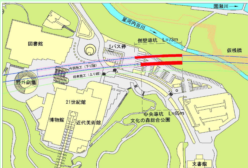
トンネル位置図 (平成17年9月30日 現在)
