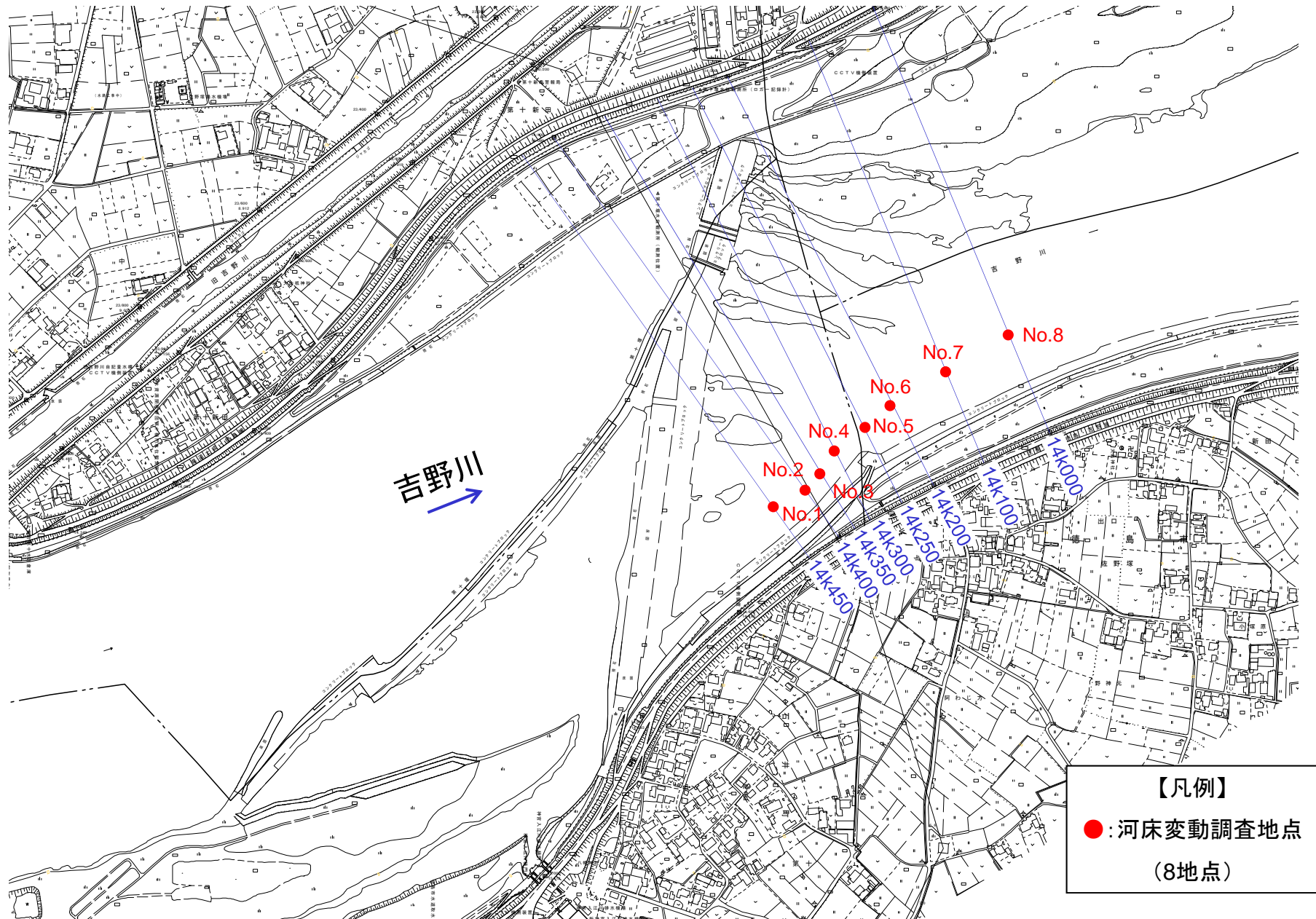
水圧計設置位置図
