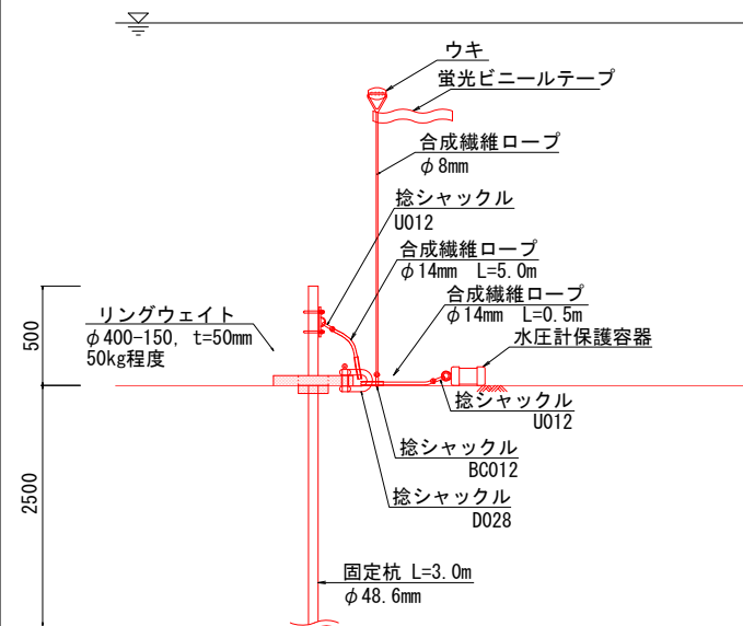
水圧計設置要領図
