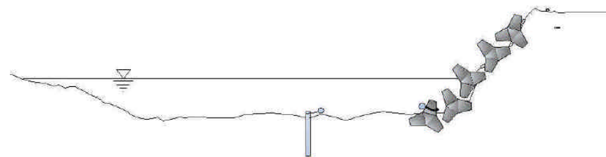
堰下流右岸深掘状況調査模式図
