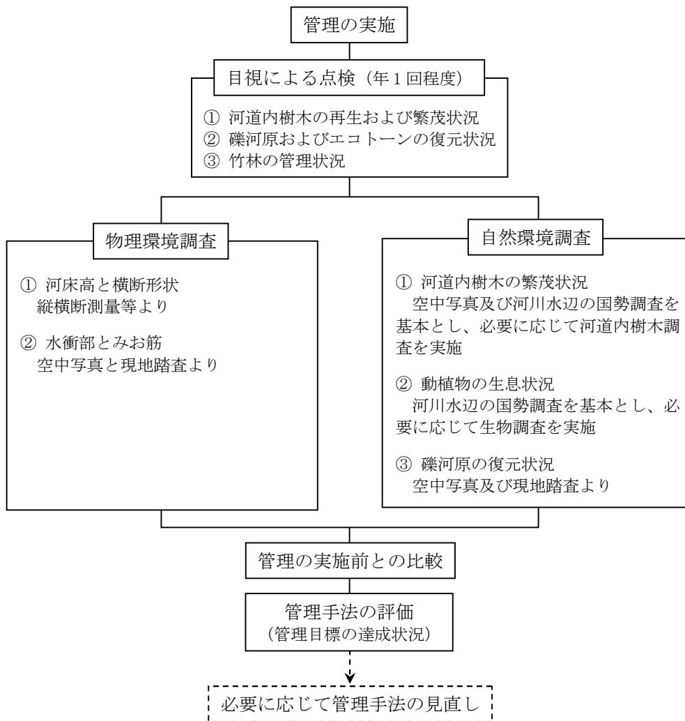
図 5.2.1 樹木管理のモニタリングフロー (案)
