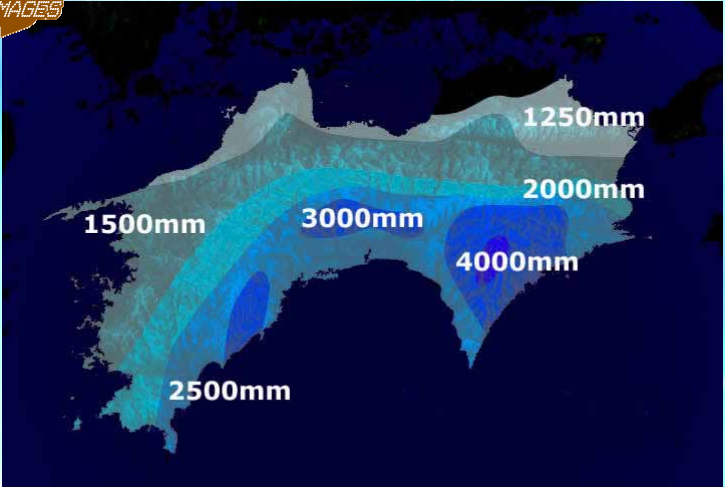
四国地方年平均降水量図
