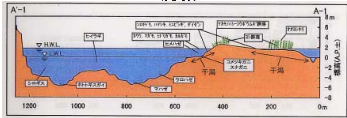
断面図
