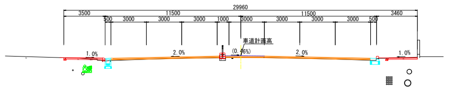
標準断面図
