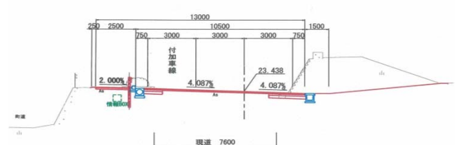
標準断面図
