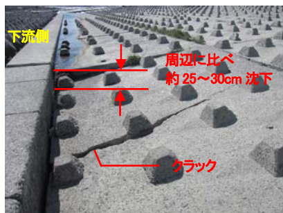
コンクリート版の損傷状況
