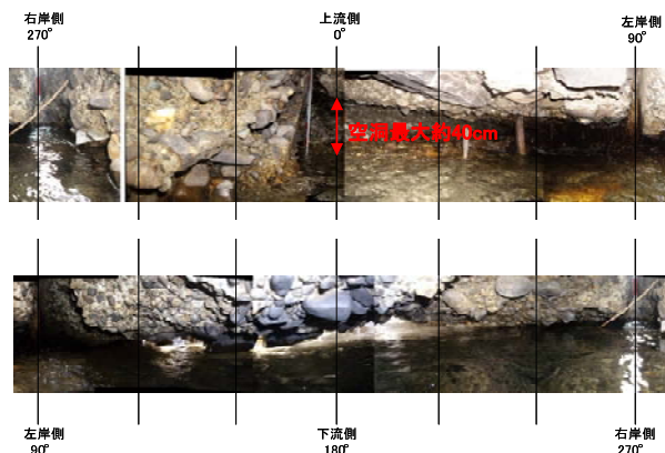
堰内部（修繕箇所）の状況
