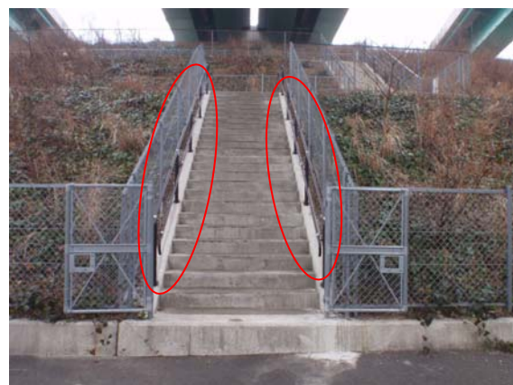
改良後: 階段部に手摺りを設置
