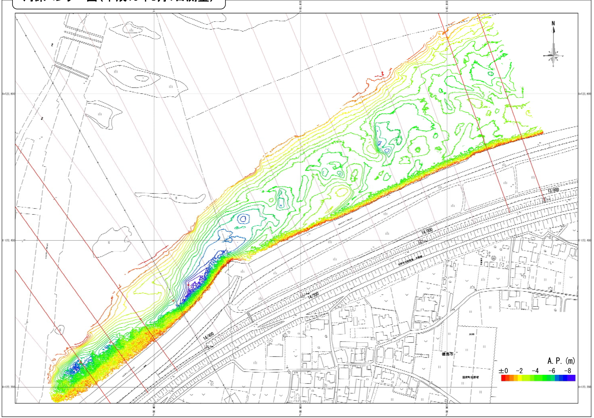
河床コンター図(平成19年8月1日測量)
