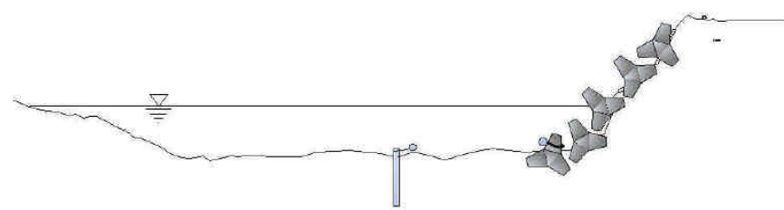
堰下流右岸深掘状況調査模式図
