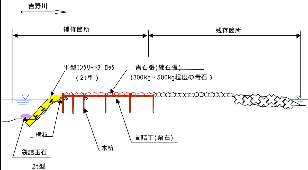
青石張 (練石張)イメージ図
