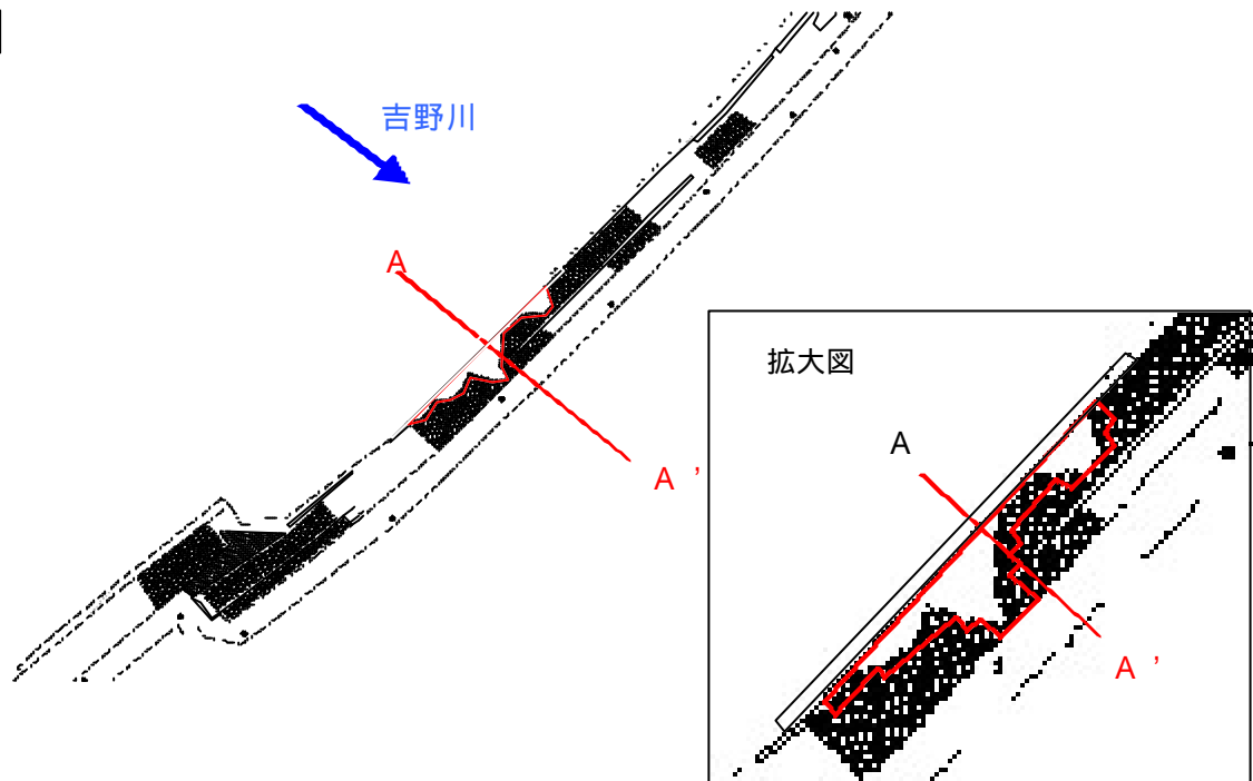
標準断面図ポンチ絵 (A - A'断面)
