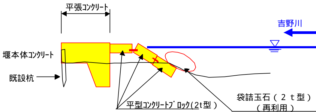
断面図A - A (ポンチ絵)
