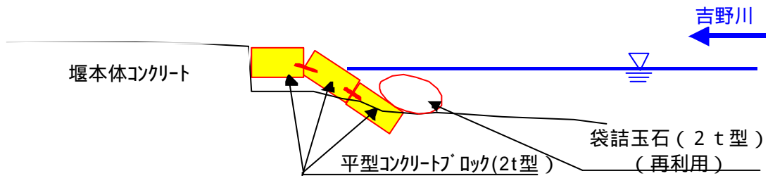
断面図B - B (ポンチ絵)
