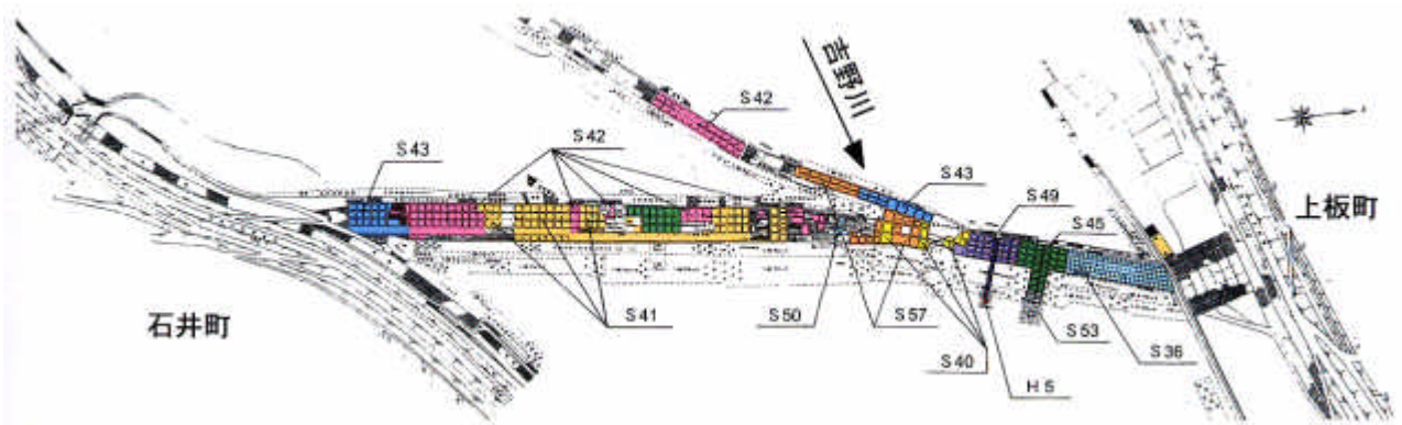
図 - 2 第十堰本体災害復旧等履歴平面図
