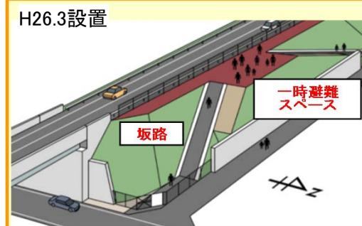
南国安芸道路に設けられた緊急避難施設
