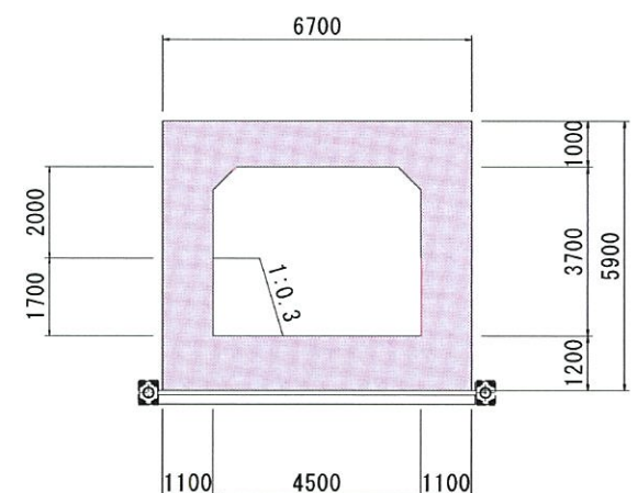
横断面図
