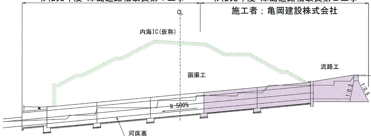
縦断面図
