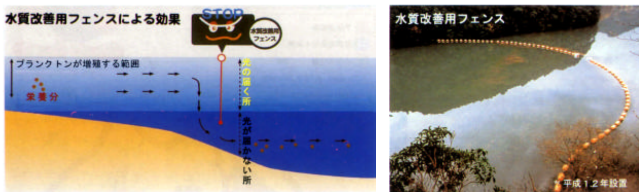
図2.2.7 プランクトンの大量発生を防ぐための水質改善用フェンスの設置(野村ダム)
