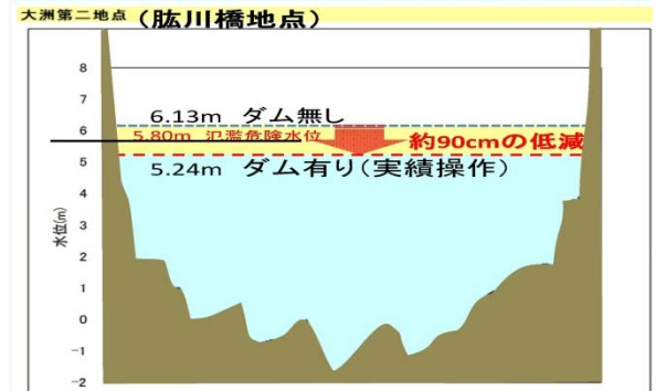
平成29年9月台風18号時に鹿野川ダムと野村ダムで連携して取り組んだ「特別防災操作」について下流水位低減効果等を報告
