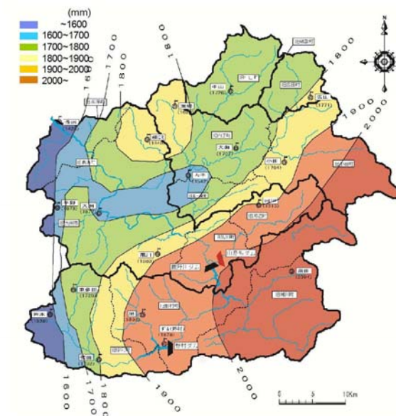
図 1.1.7 肱川流域の年平均降水量分布図
