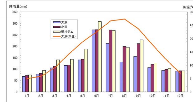
図 1.1.6 肱川流域における降水量および気温の月平均値
