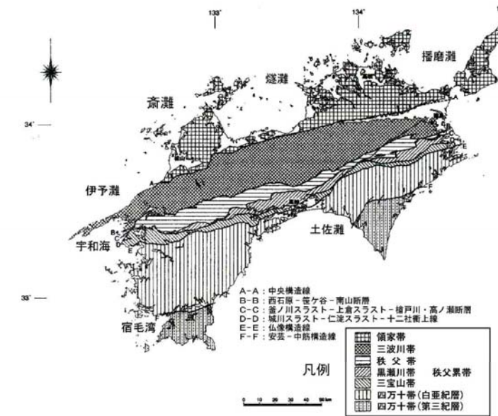
図 1.1.4 四国地質概略図
