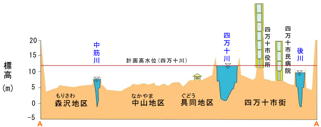
図1.2.2 中村平野と洪水時における四万十川の水面との関係 (A-A' 断面) (地盤標高と計画高水位との比較)
