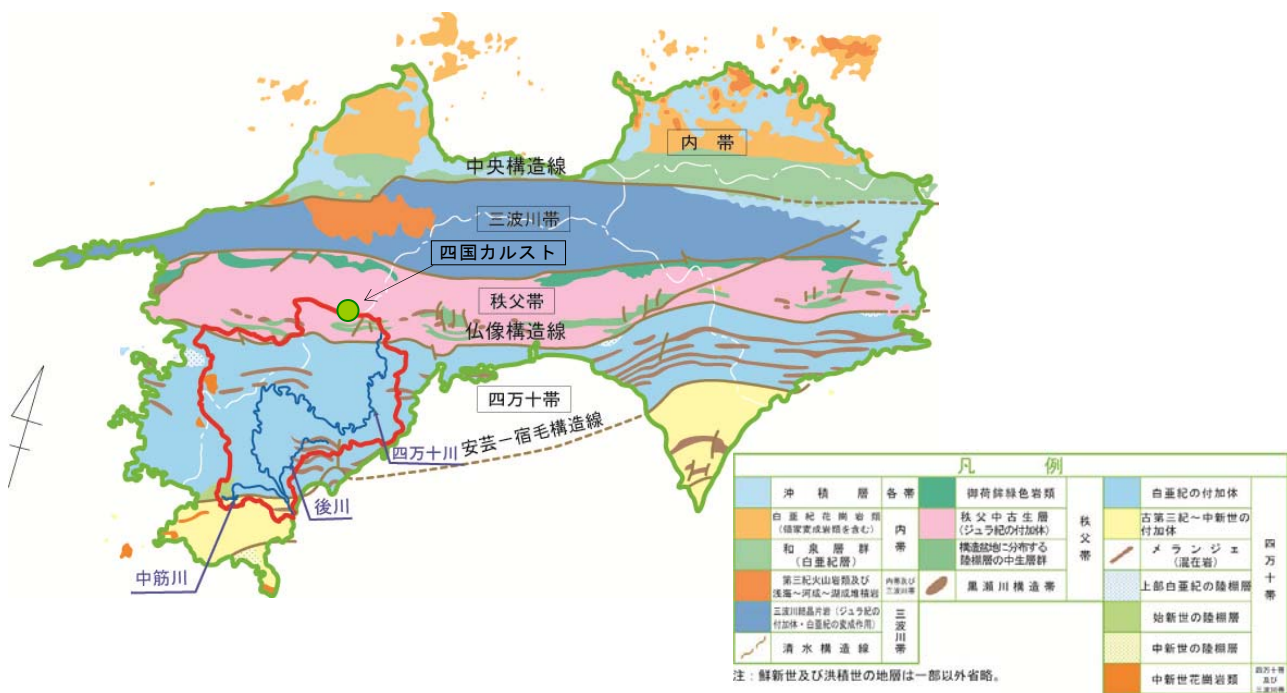
図1.3.1 四国の地質分布図
