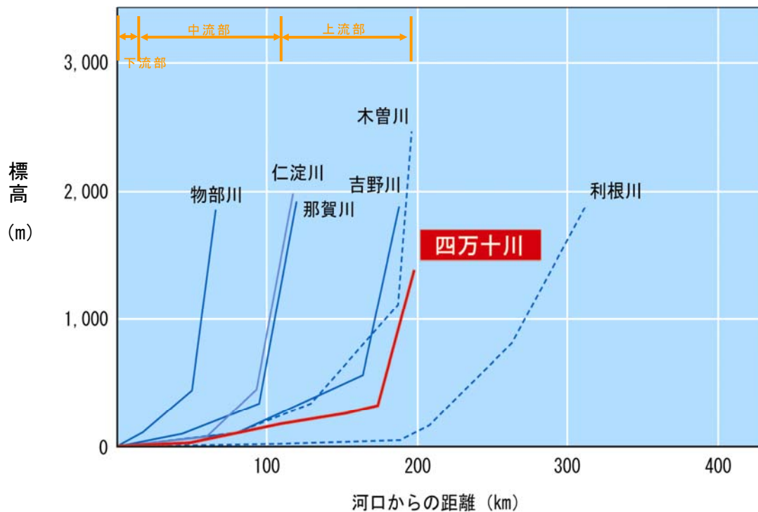
図1.2.3 河床勾配の比較図 (四万十川と他河川)
