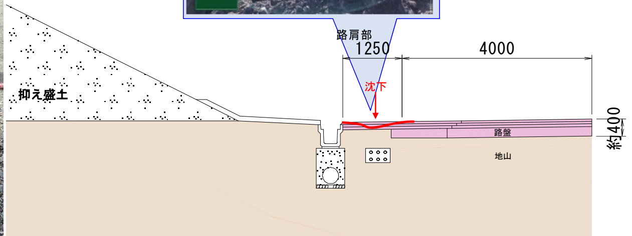
【断面図】
