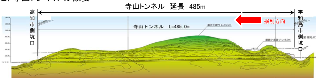
トンネル断面図
