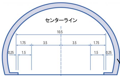
トンネル断面図
