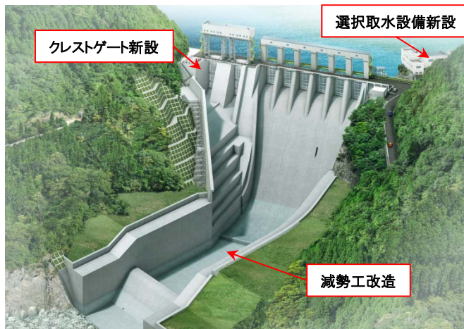
長安口ダム改造イメージ
