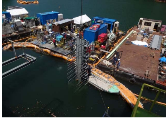
側部戸当り設置作業状況
