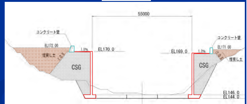
C-C断面
