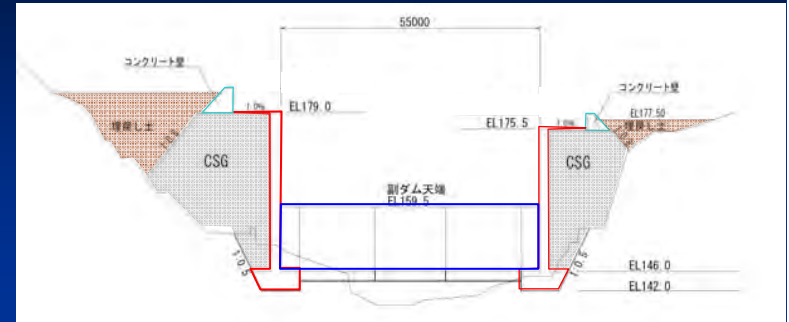
B-B断面
